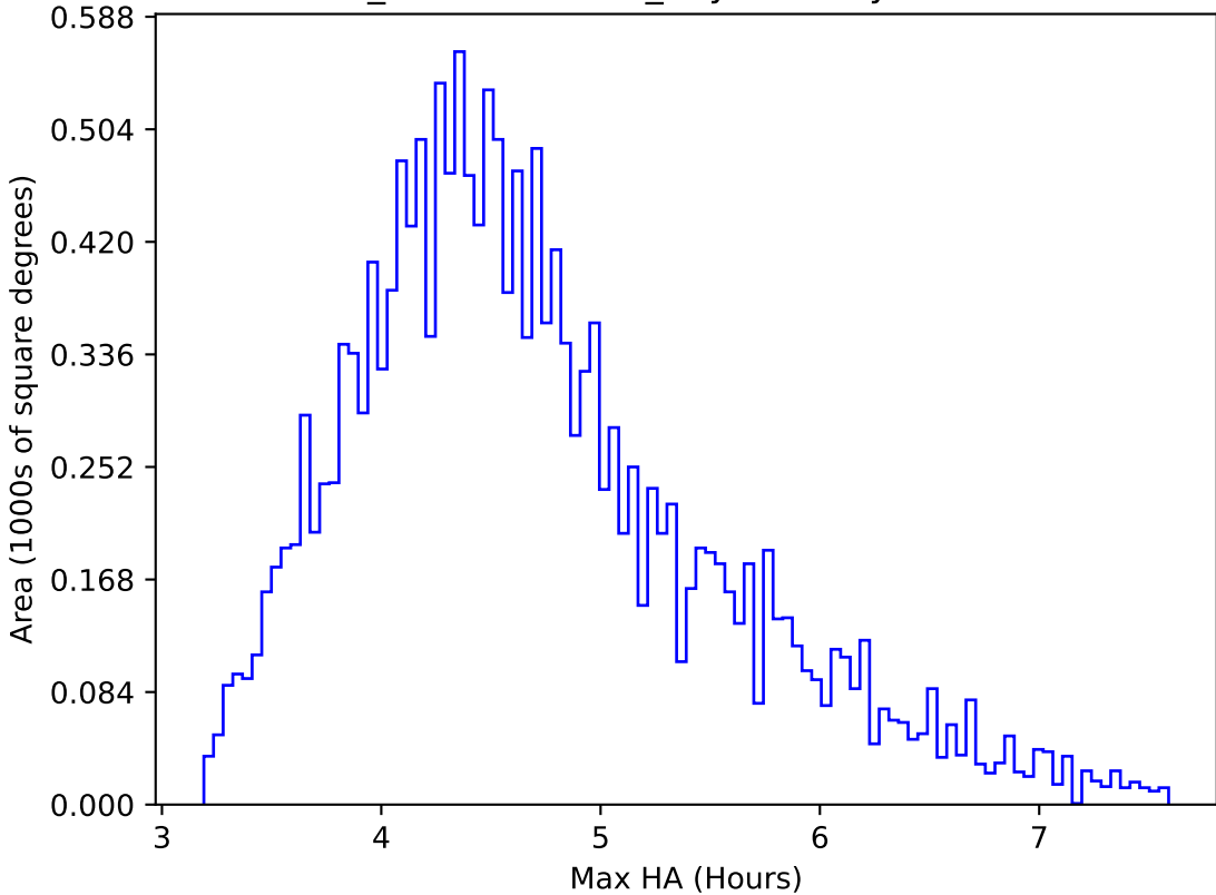
weather_cloudso31v3.4_10yrs WFD y band: Max HA
