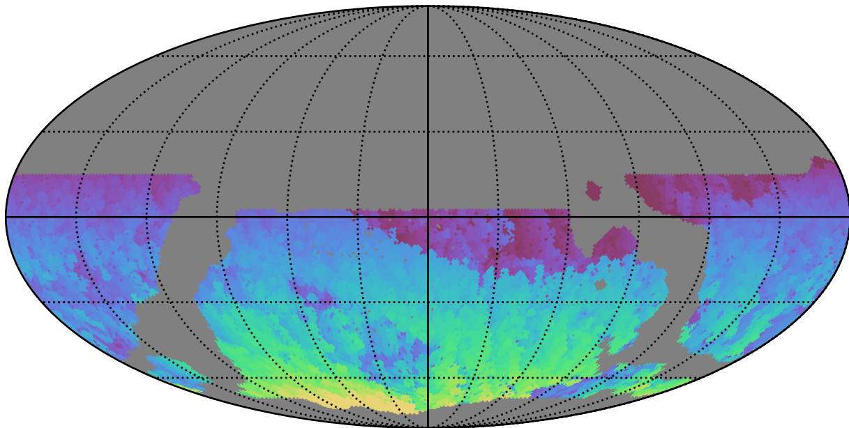
weather_cloudso31v3.4_10yrs WFD i band: Max HA
