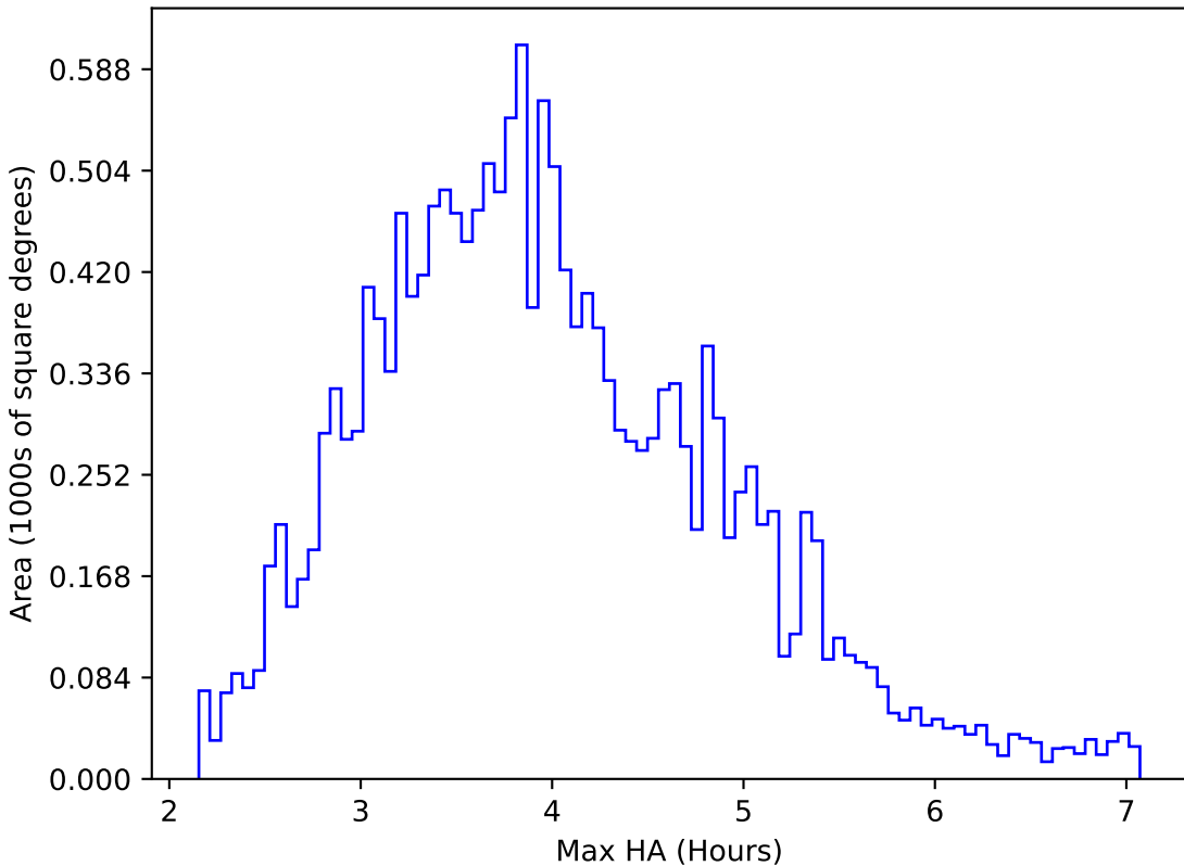
weather_cloudso31v3.4_10yrs WFD g band: Max HA
