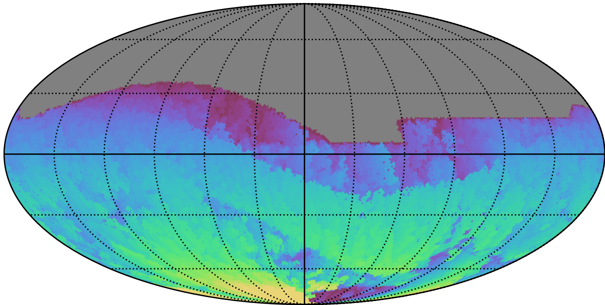
weather_cloudso31v3.4_10yrs All sky z band: Max HA
