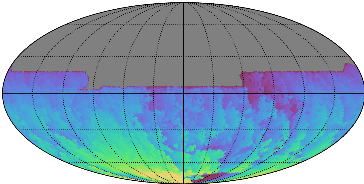
weather_cloudso31v3.4_10yrs All sky y band: Max HA
