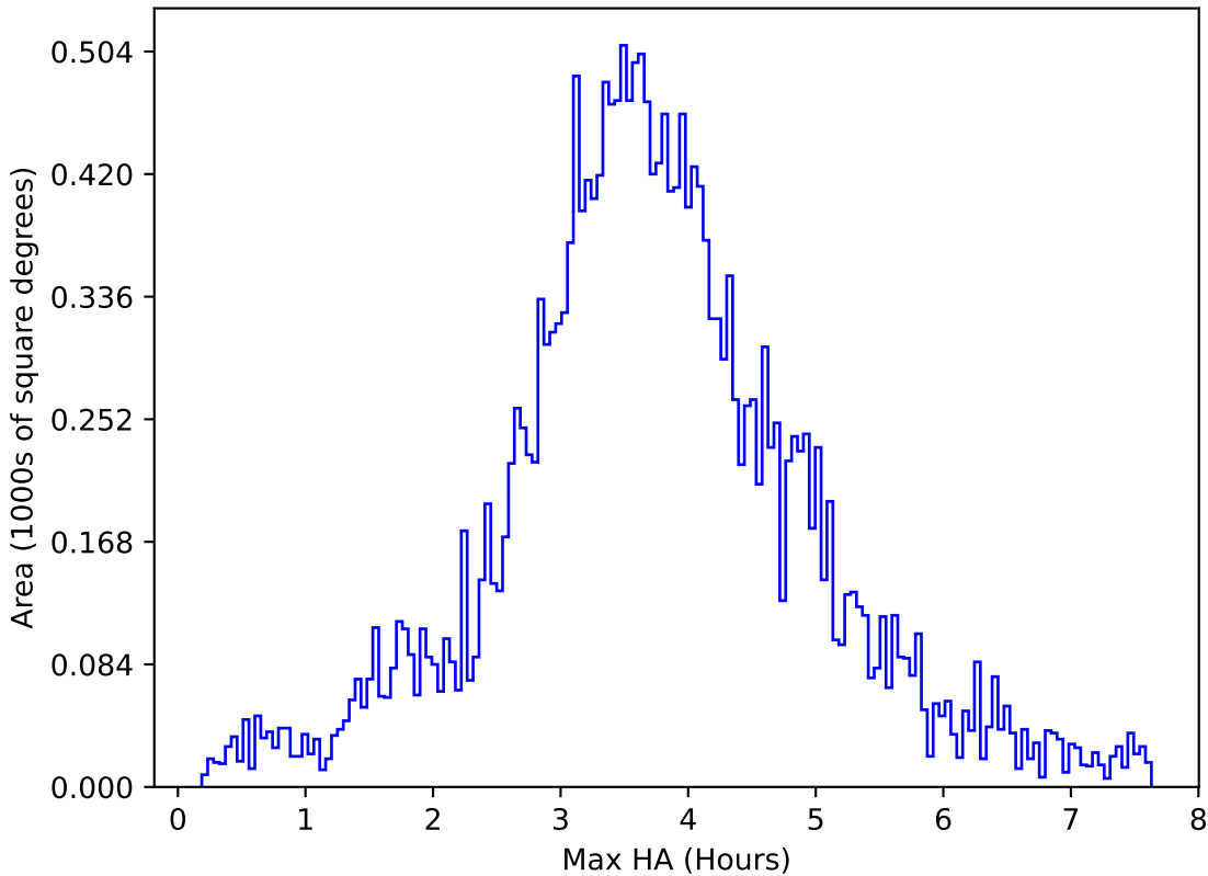
weather_cloudso31v3.4_10yrs All sky u band: Max HA
