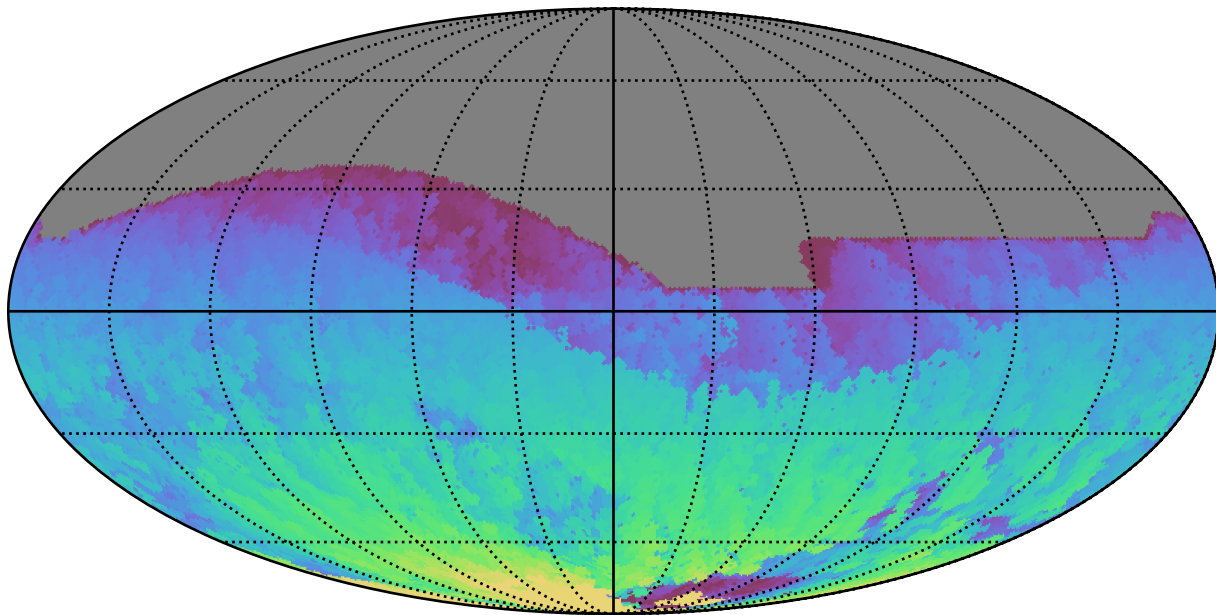
weather_cloudso31v3.4_10yrs All sky i band: Max HA
