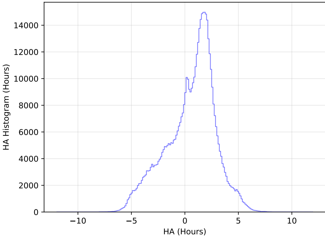
weather_cloudso31v3.4_10yrs WFD i band: HA Histogram
