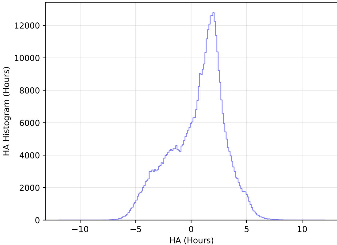
weather_cloudso31v3.4_10yrs All sky z band: HA Histogram
