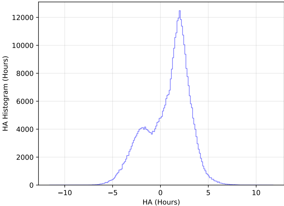
weather_cloudso31v3.4_10yrs All sky y band: HA Histogram
