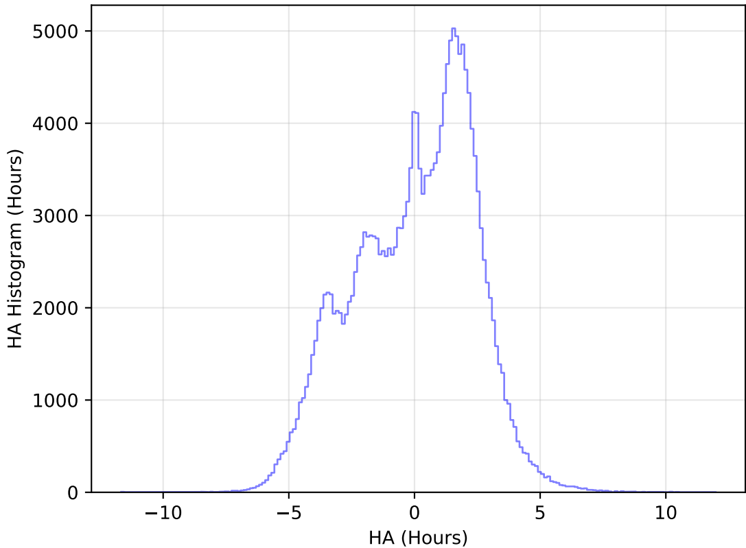
weather_cloudso31v3.4_10yrs All sky g band: HA Histogram
