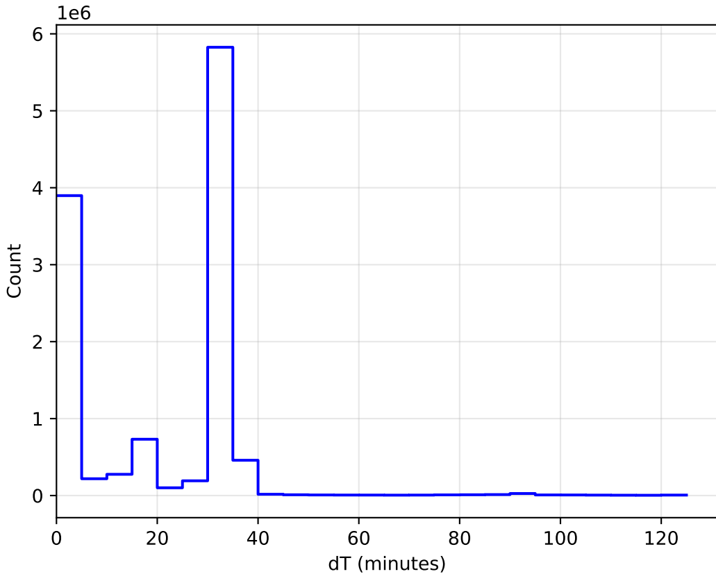
weather_cloudso31v3.4_10yrs WFD: DeltaT Histogram
