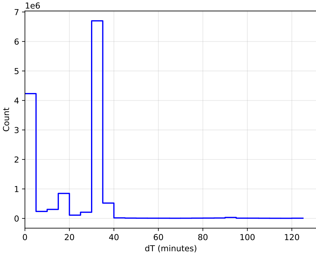
weather_cloudso31v3.4_10yrs All sky: DeltaT Histogram
