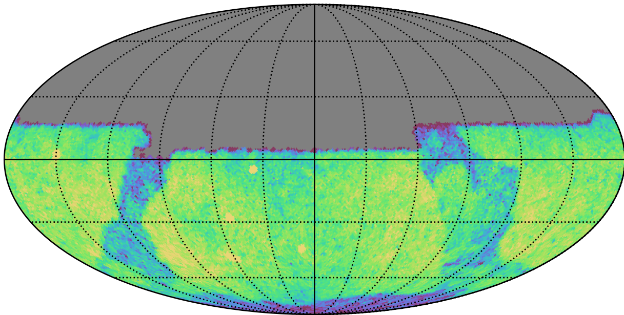
weather_cloudso31v3.4_10yrs Yr 1 y band: CoaddM5
