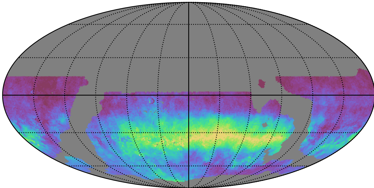
weather_cloudso31v3.4_10yrs WFD i band: AngleRms rotSkyPos
