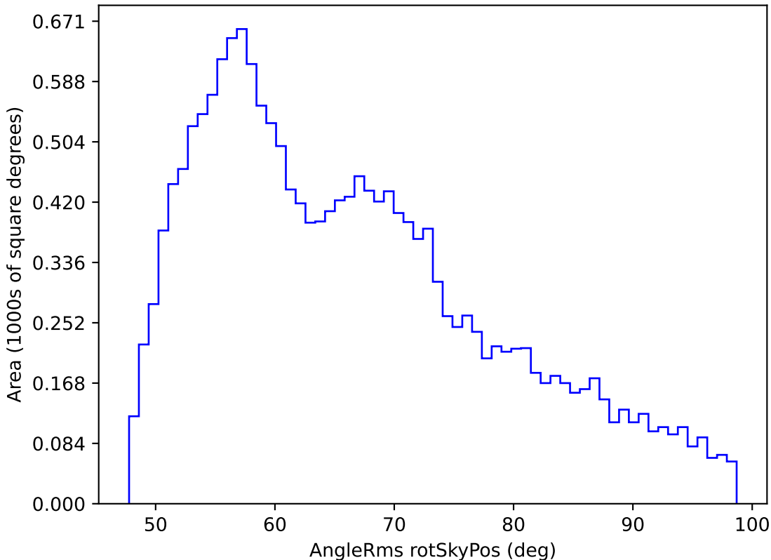
weather_cloudso31v3.4_10yrs WFD i band: AngleRms rotSkyPos
