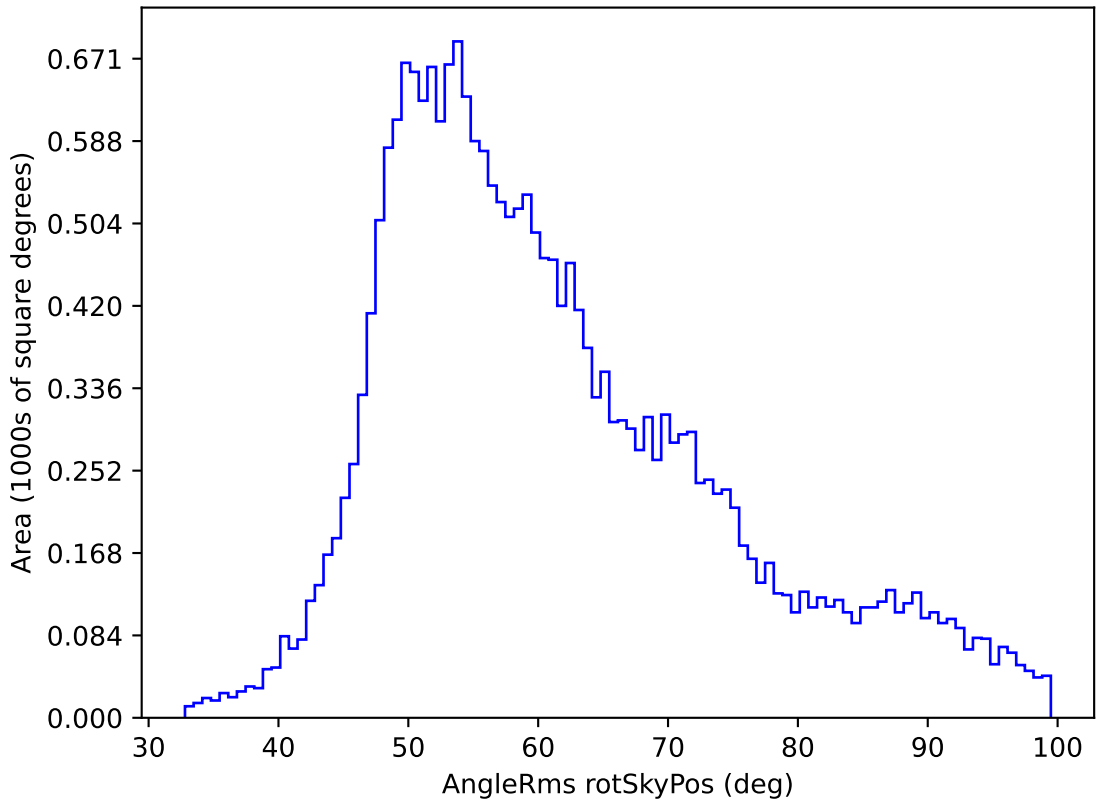
weather_cloudso31v3.4_10yrs All sky y band: AngleRms rotSkyPos
