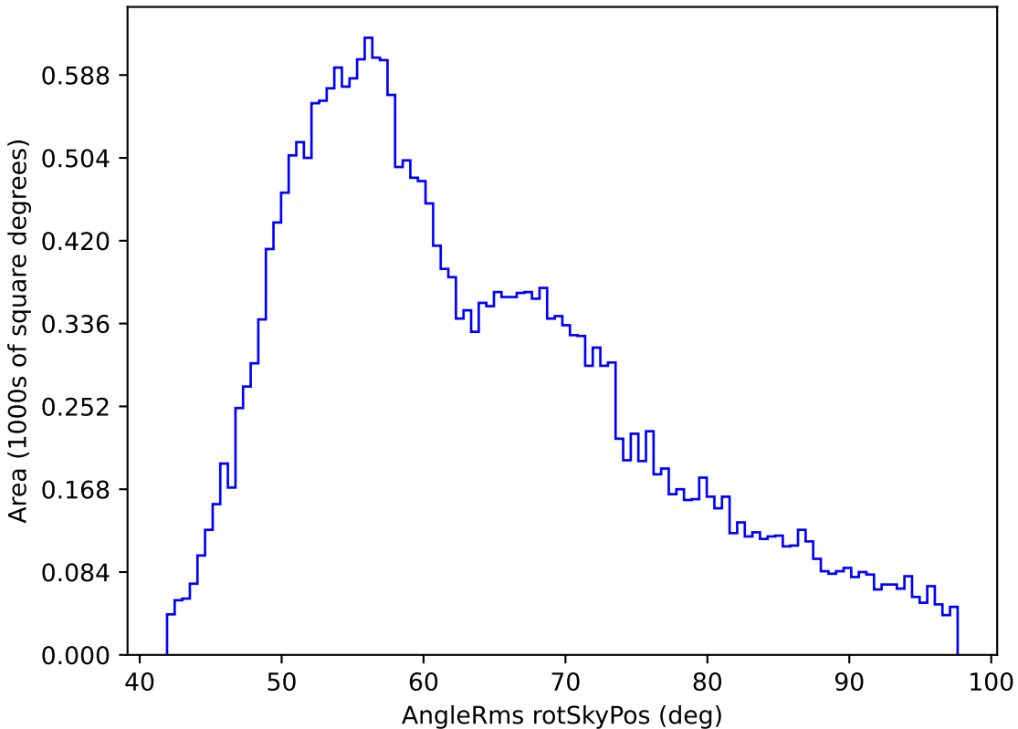
weather_cloudso31v3.4_10yrs All sky i band: AngleRms rotSkyPos
