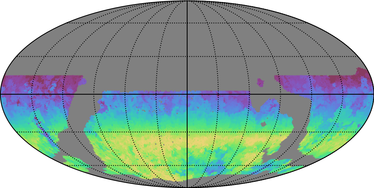
weather_cloudso31v3.4_10yrs WFD z band: AngleRange rotSkyPos
