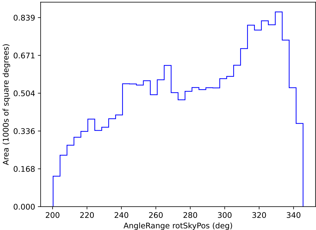
weather_cloudso31v3.4_10yrs WFD r band: AngleRange rotSkyPos
