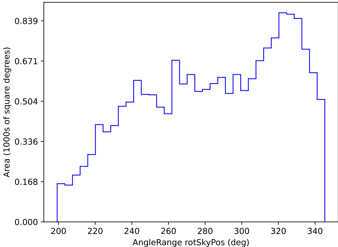
weather_cloudso31v3.4_10yrs WFD i band: AngleRange rotSkyPos
