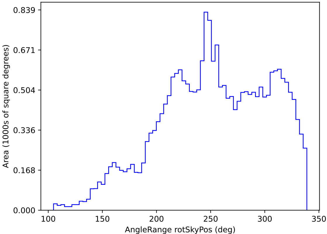
weather_cloudso31v3.4_10yrs All sky y band: AngleRange rotSkyPos
