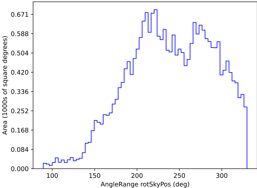
weather_cloudso31v3.4_10yrs All sky u band: AngleRange rotSkyPos
