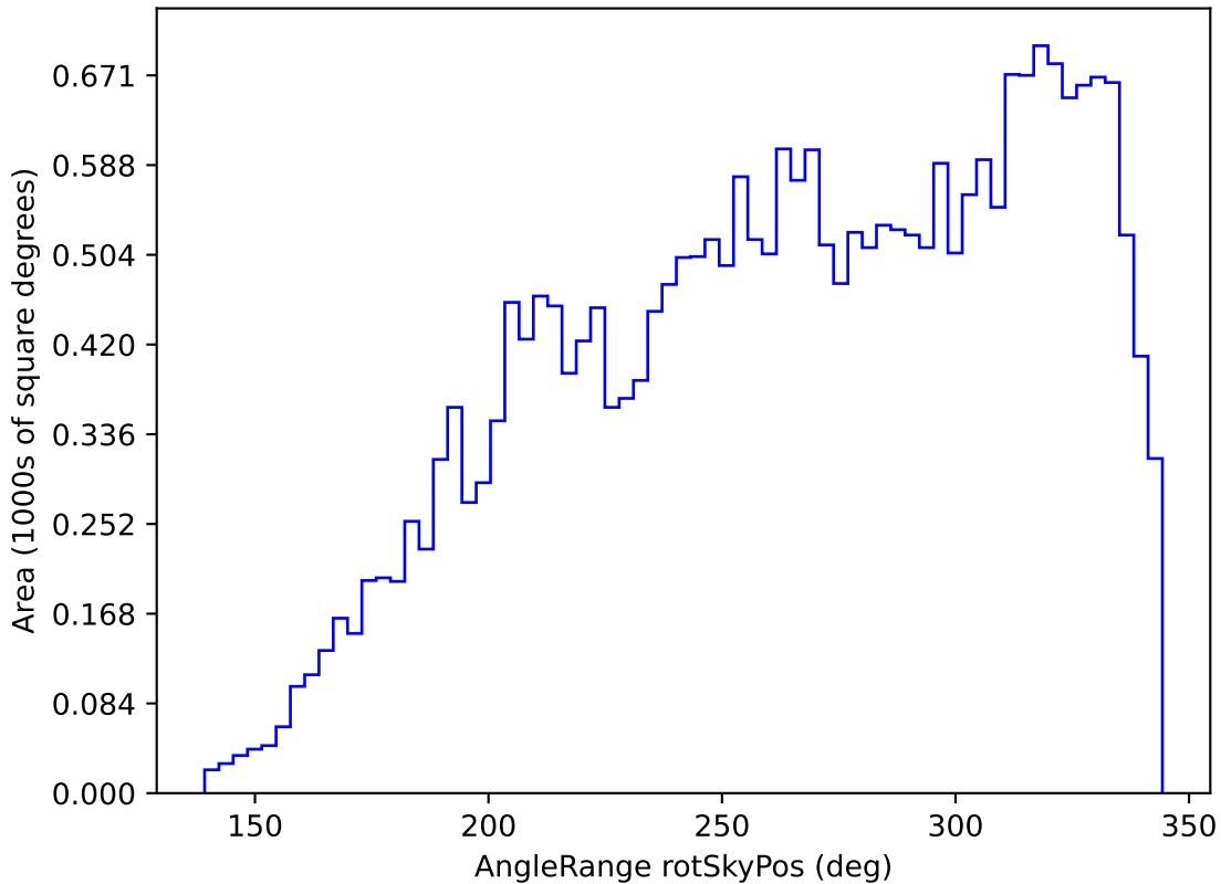
weather_cloudso31v3.4_10yrs All sky r band: AngleRange rotSkyPos
