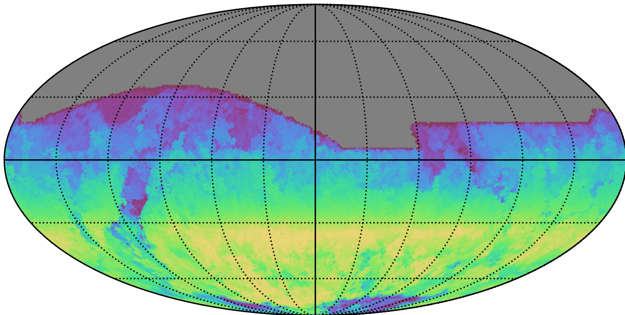
weather_cloudso31v3.4_10yrs All sky i band: AngleRange rotSkyPos
