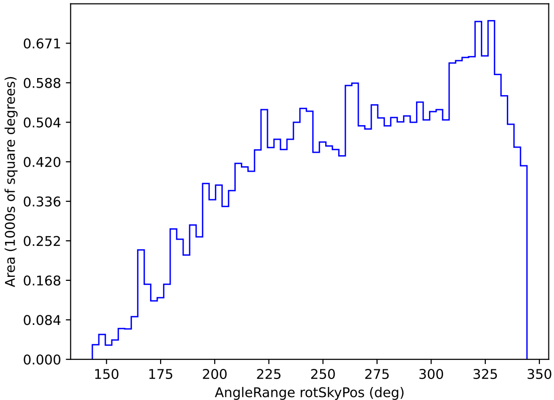
weather_cloudso31v3.4_10yrs All sky i band: AngleRange rotSkyPos
