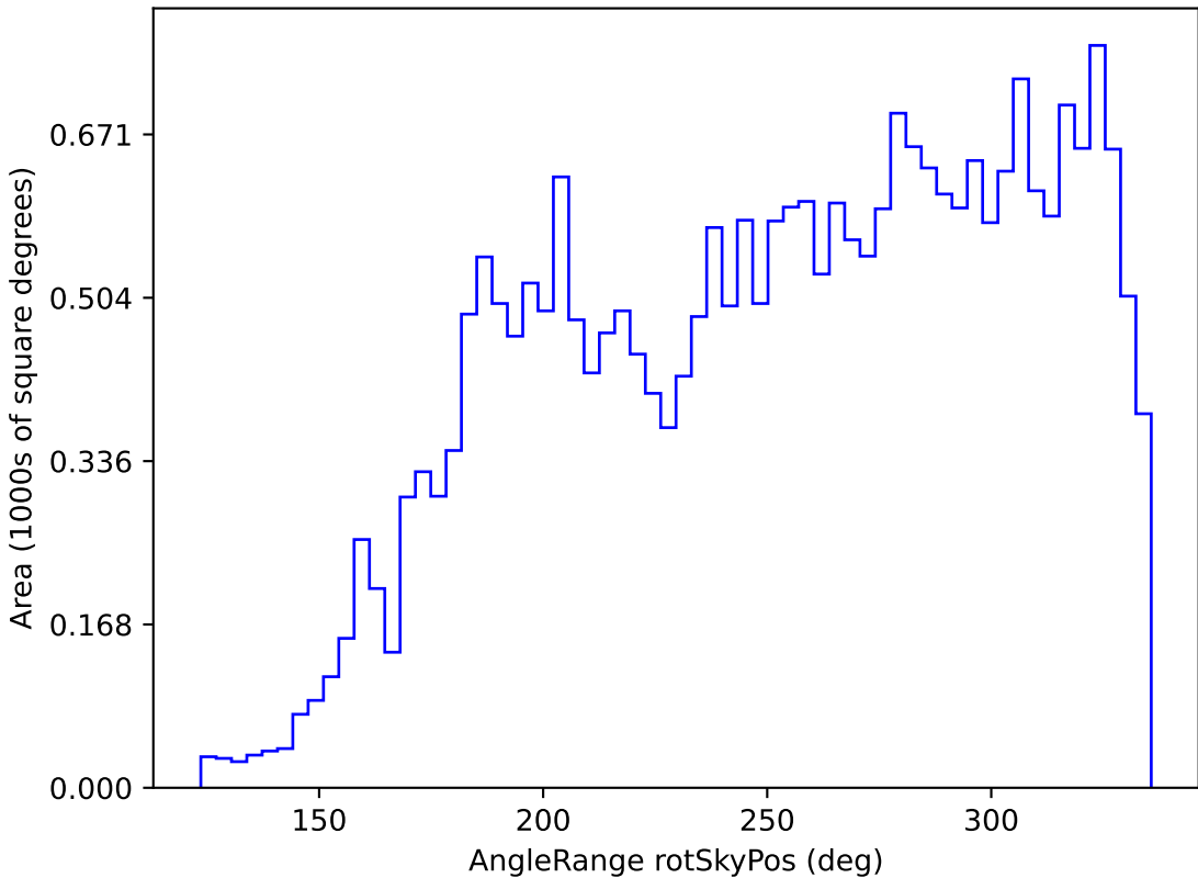
weather_cloudso31v3.4_10yrs All sky g band: AngleRange rotSkyPos
