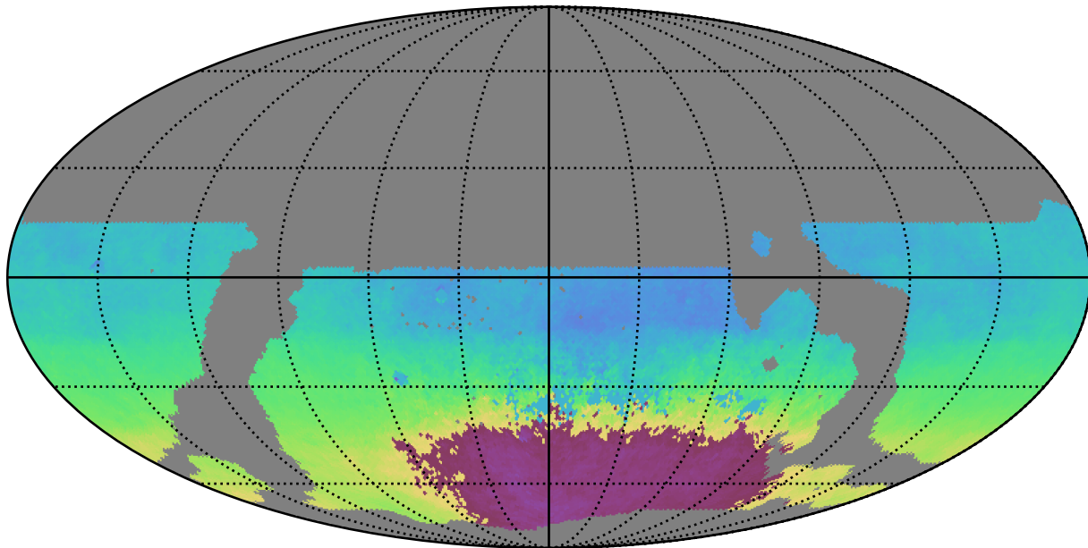
weather_cloudso31v3.4_10yrs WFD y band: AngleMean rotSkyPos
