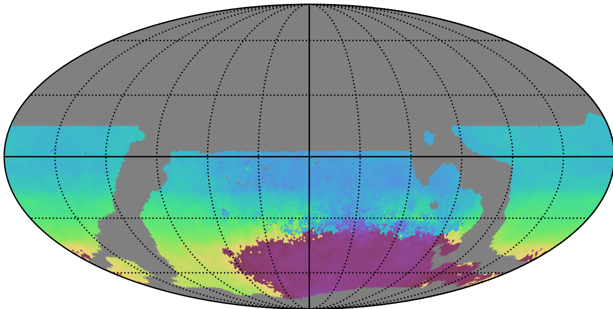
weather_cloudso31v3.4_10yrs WFD r band: AngleMean rotSkyPos
