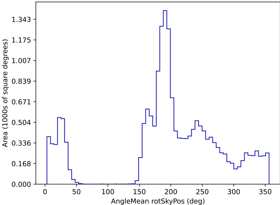
weather_cloudso31v3.4_10yrs WFD i band: AngleMean rotSkyPos
