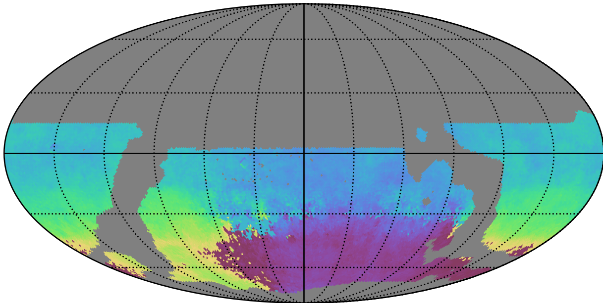
weather_cloudso31v3.4_10yrs WFD g band: AngleMean rotSkyPos
