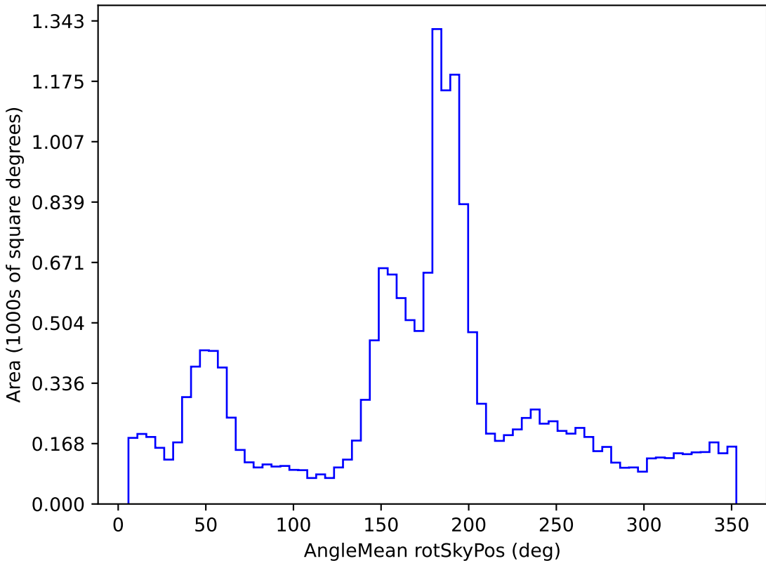
weather_cloudso31v3.4_10yrs WFD g band: AngleMean rotSkyPos
