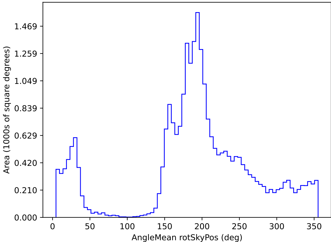
weather_cloudso31v3.4_10yrs All sky z band: AngleMean rotSkyPos
