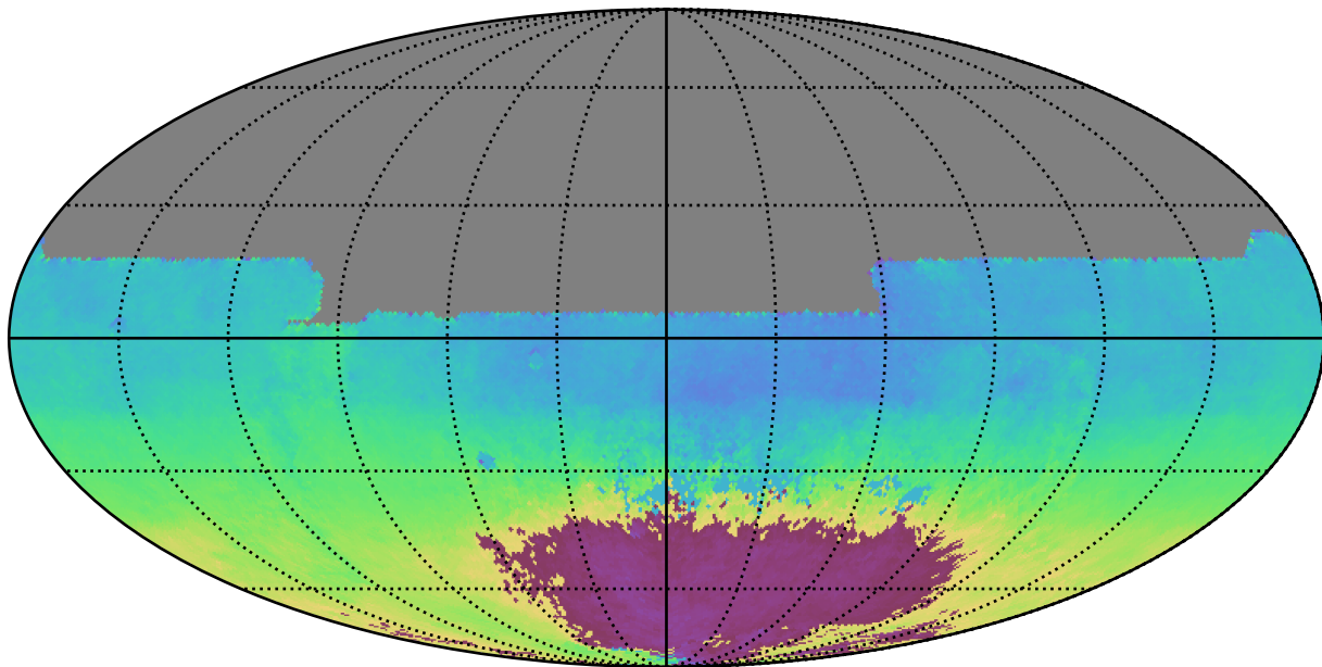
weather_cloudso31v3.4_10yrs All sky y band: AngleMean rotSkyPos
