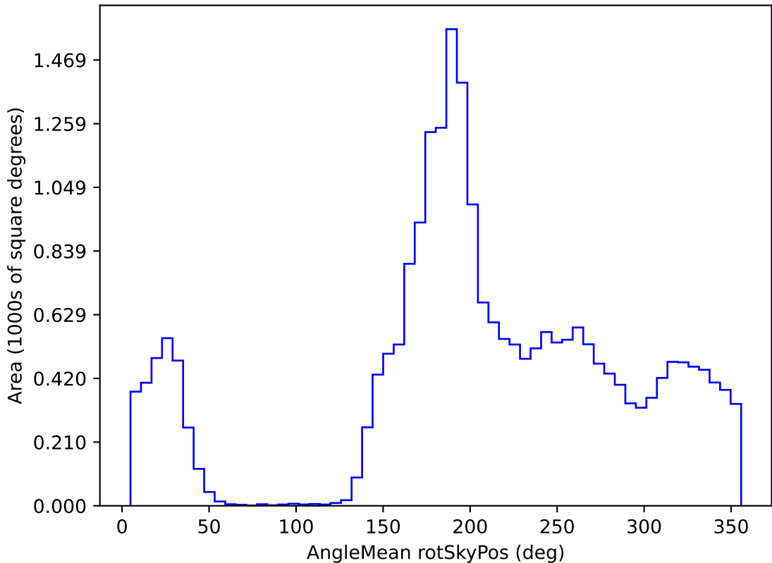
weather_cloudso31v3.4_10yrs All sky y band: AngleMean rotSkyPos
