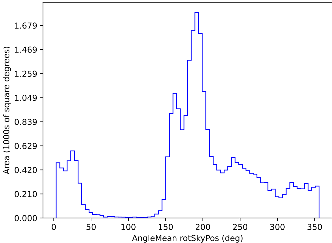
weather_cloudso31v3.4_10yrs All sky i band: AngleMean rotSkyPos
