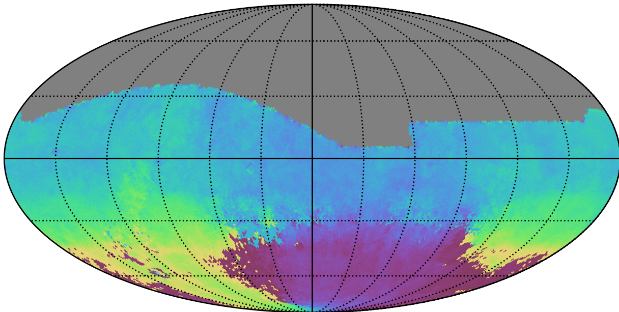
weather_cloudso31v3.4_10yrs All sky g band: AngleMean rotSkyPos
