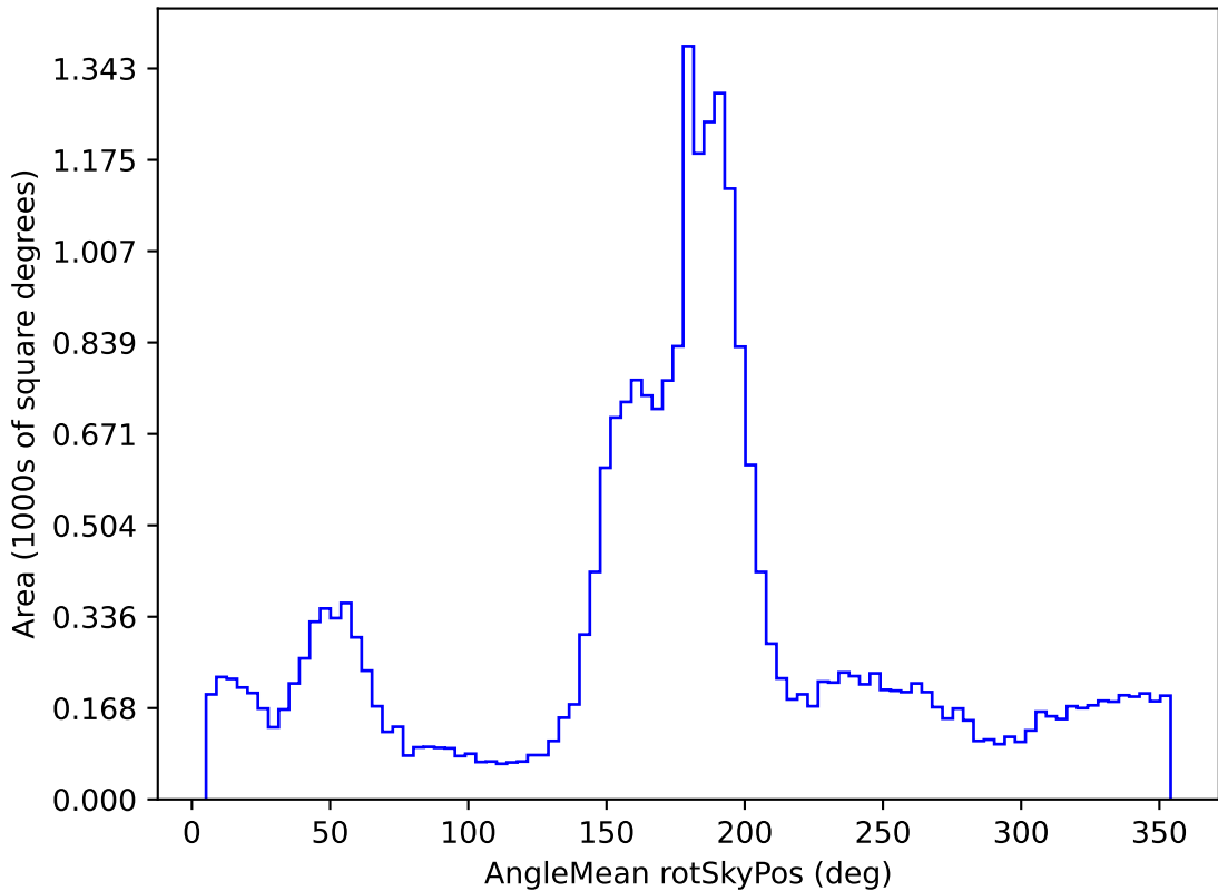
weather_cloudso31v3.4_10yrs All sky g band: AngleMean rotSkyPos
