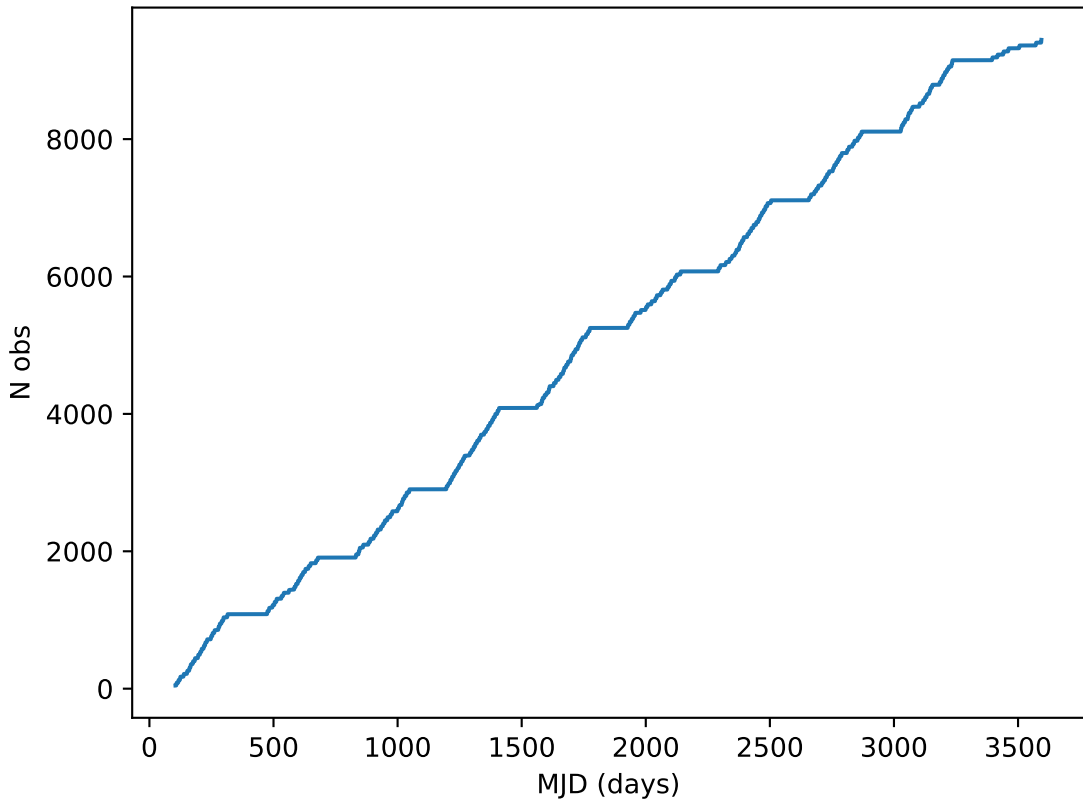
weather_cloudso31v3.4_10yrs note like DD:EDFS_a%: Cumulative
