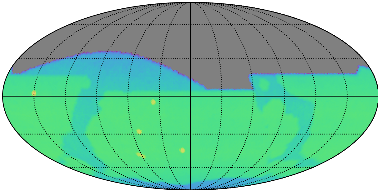
weather_cloudso31v3.4_10yrs i: CoaddM5
