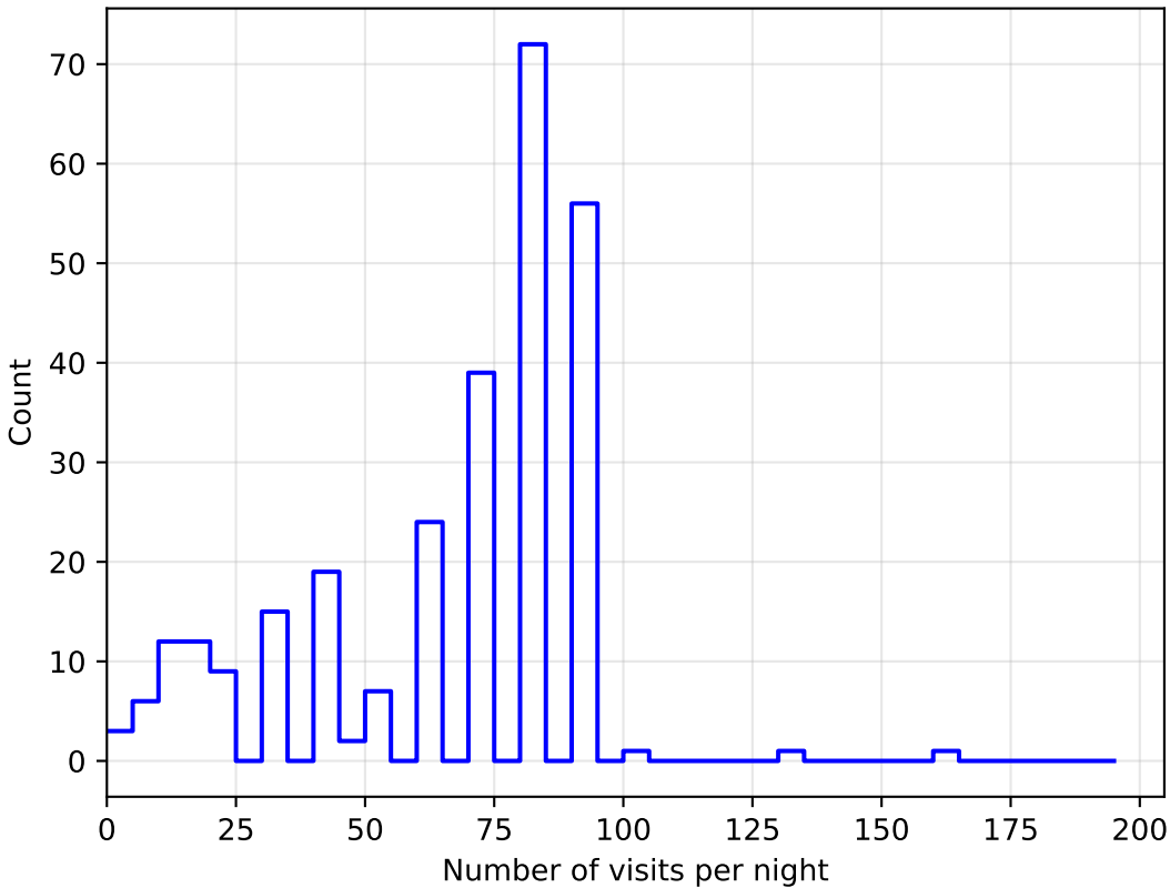
weather_cloudso31v3.4_10yrs all bands: DD:XMM_LSS NVisitsPerNight
