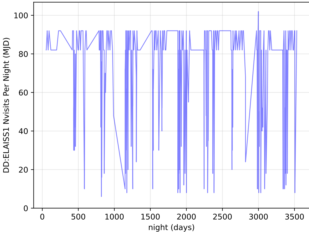
weather_cloudso31v3.4_10yrs all bands: DD:ELAISS1 Nvisits Per Night
