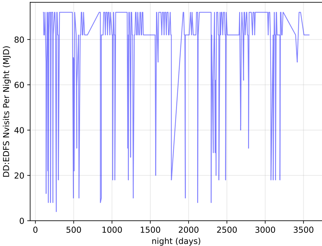
weather_cloudso31v3.4_10yrs all bands: DD:EDFS Nvisits Per Night
