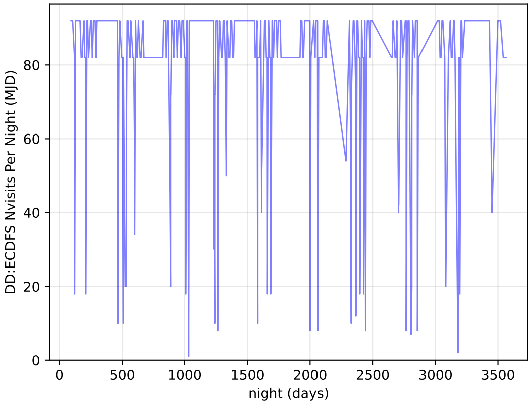
weather_cloudso31v3.4_10yrs all bands: DD:ECDFS Nvisits Per Night
