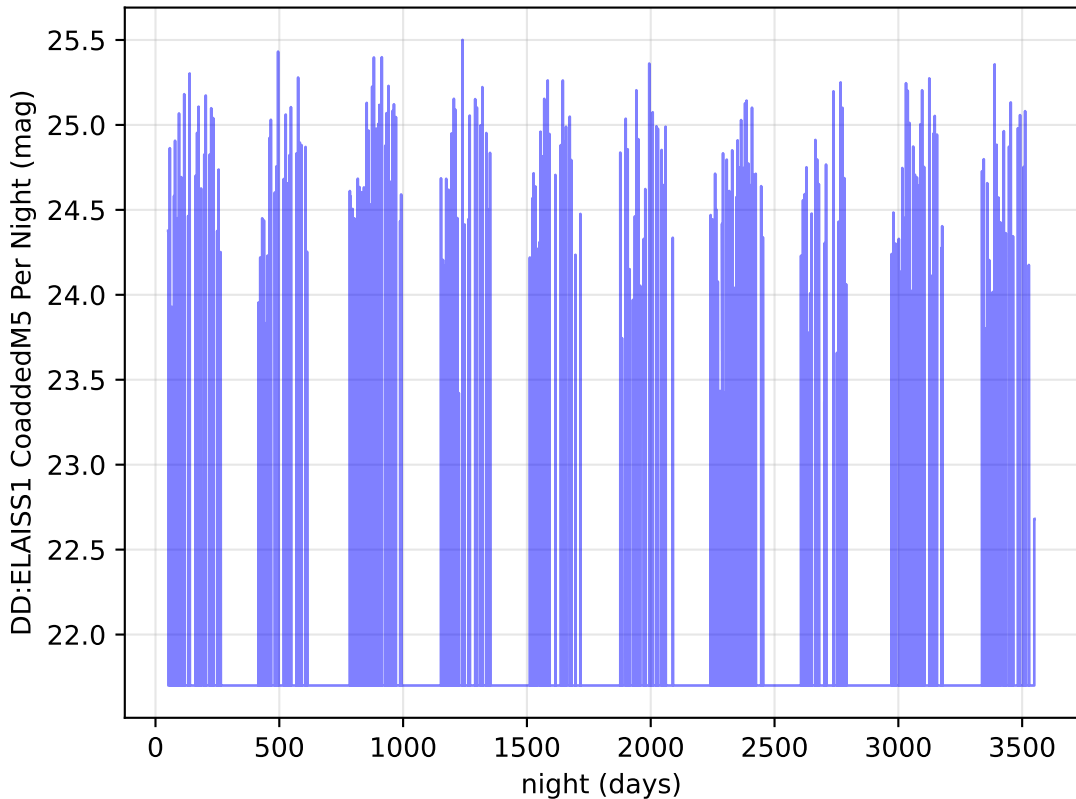
weather_cloudso30v3.5_10yrs z band: DD:ELAISS1 CoaddedM5 Per Night
