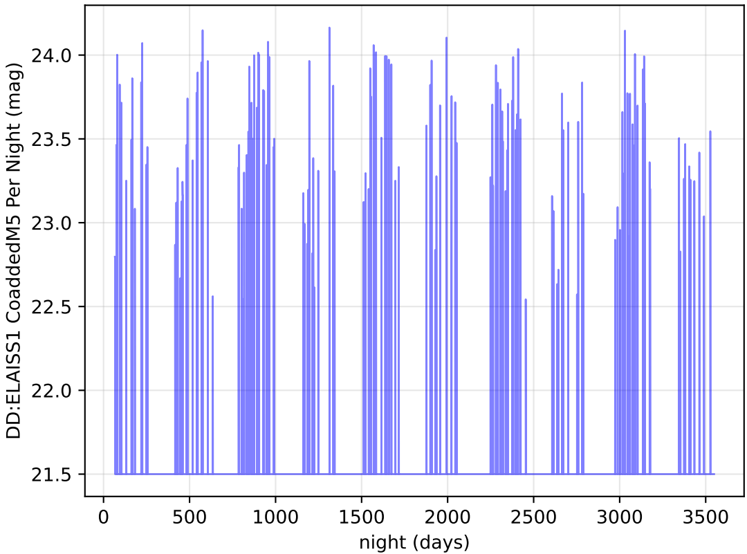
weather_cloudso30v3.5_10yrs y band: DD:ELAISS1 CoaddedM5 Per Night
