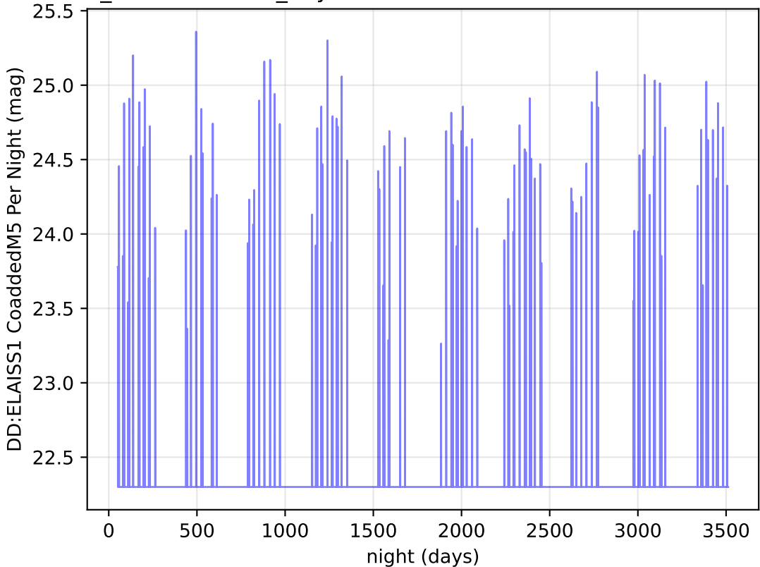
weather_cloudso30v3.5_10yrs u band: DD:ELAISS1 CoaddedM5 Per Night
