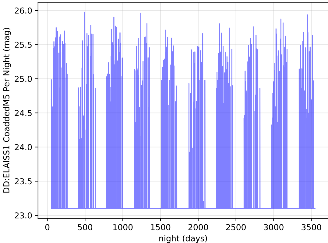
weather_cloudso30v3.5_10yrs i band: DD:ELAISS1 CoaddedM5 Per Night
