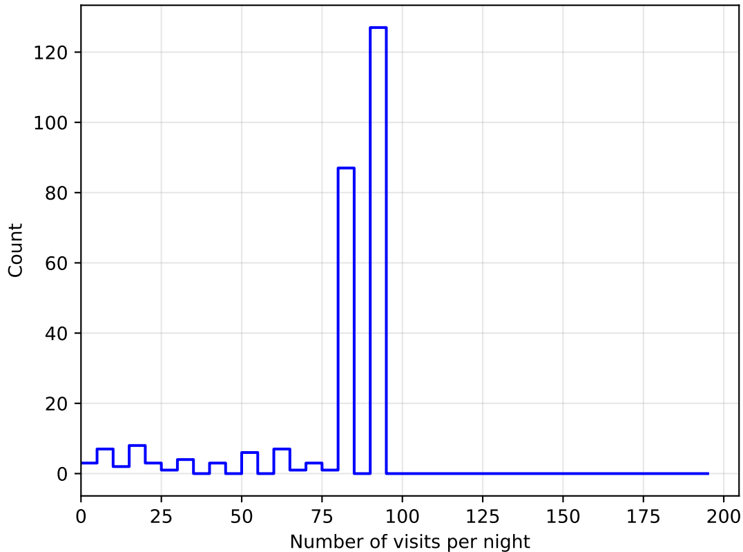
weather_cloudso30v3.5_10yrs all bands: DD:EDFS NVisitsPerNight
