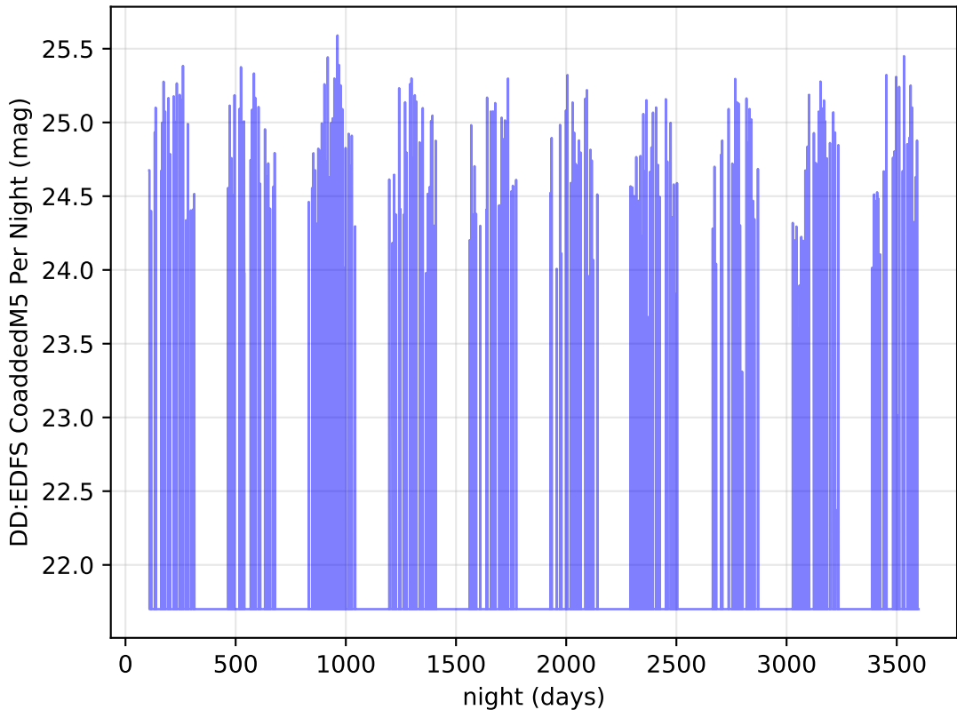
weather_cloudso30v3.5_10yrs z band: DD:EDFS CoaddedM5 Per Night
